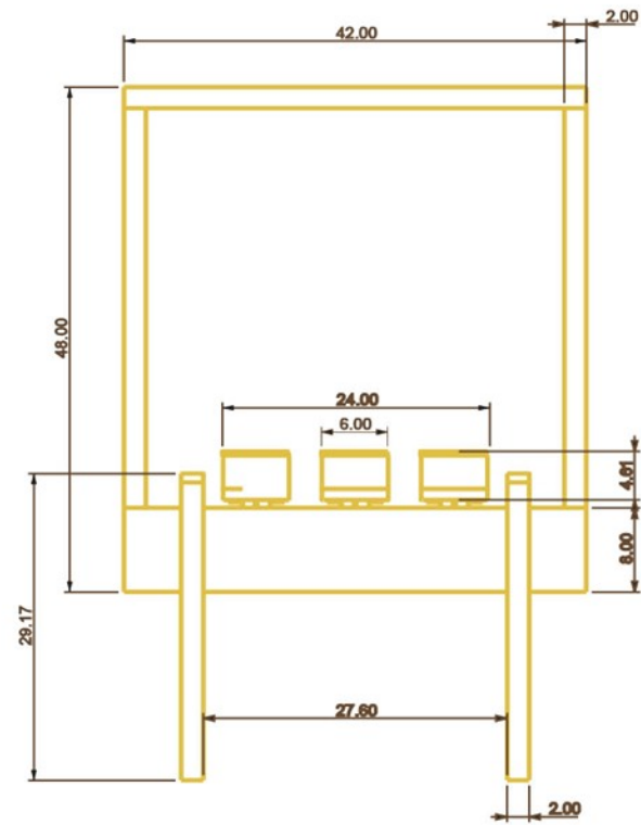
ELEVATION
